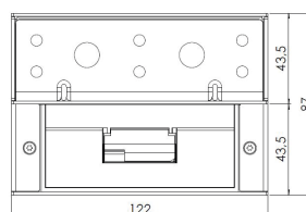
Måttskiss STEP 8 med vinkelkonsoll.
