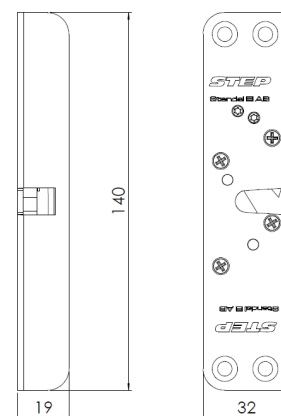
Målsatt tegning STEP 35 med vinklet stolpe.
