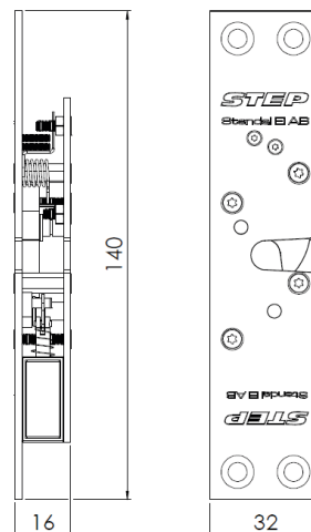
Målsatt tegning STEP 35 med plan stolpe.
