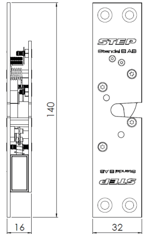
Måttskiss STEP 35 med plan stolpe.
