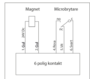
Kopplingschema.
