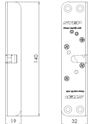
Måttskiss STEP 35 med vinklad stolpe.
