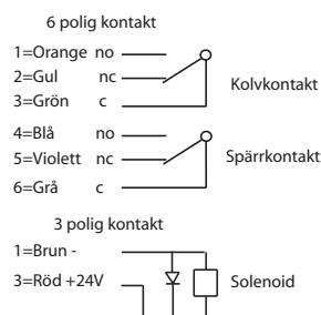
Kopplingschema med kolvkontakt.
