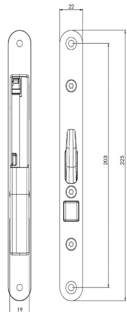
Målsatt tegning for STEP 552.
