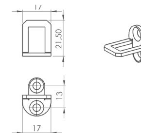
Måttskiss låsbleck
