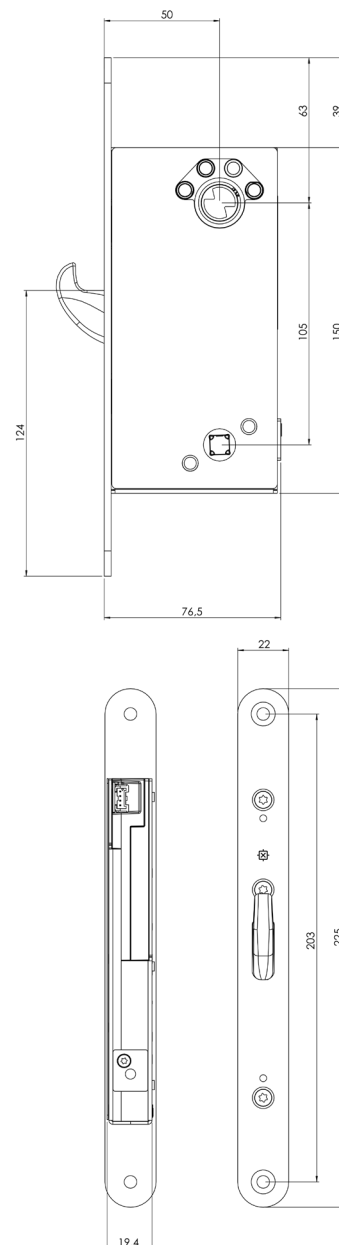
Måttskiss för STEP 351S.
