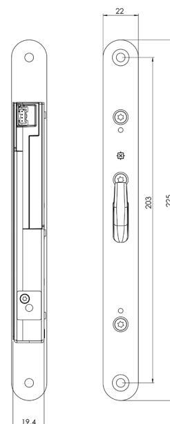
Måttskiss för STEP 351.
