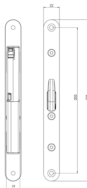
Måttkiss för STEP 551.
