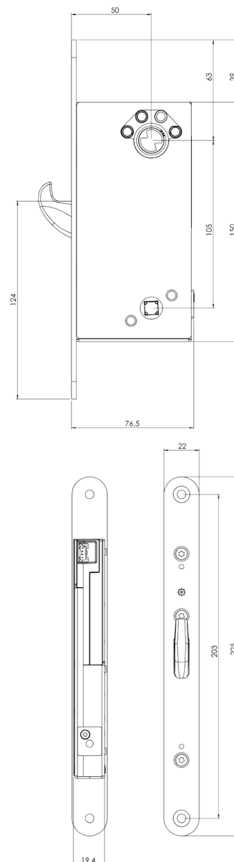
Målskitse STEP 351S.
